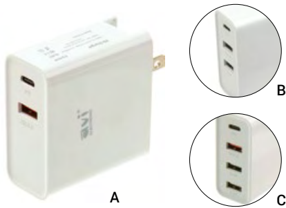
LM06-2008 PD+QC3.0 Wall Charger Input: AC 110-240V Output: A: PD+QC 48W B: PD+QC+USB 2.0 48W C: PD+QC+2*USB 2.0 48W
